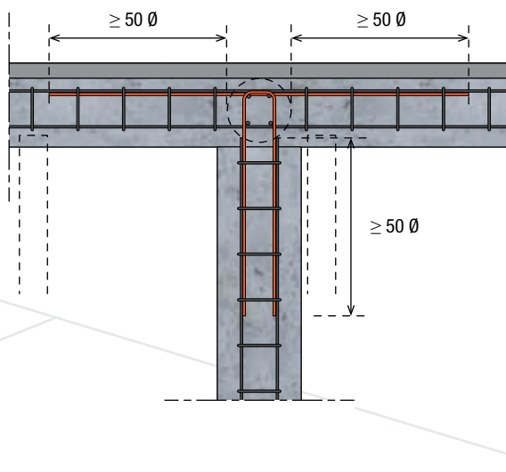
Liaison en partie courante avec boucles
