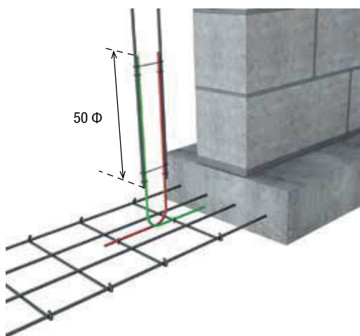
Exemples de continuité des armatures de la fondation avec un chaînage vertical en zone courante et non courante
