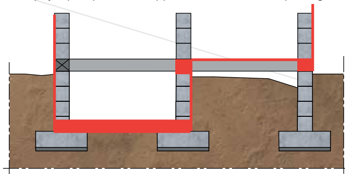
Protection contre les termites – Schéma de principe avec barrière continue
