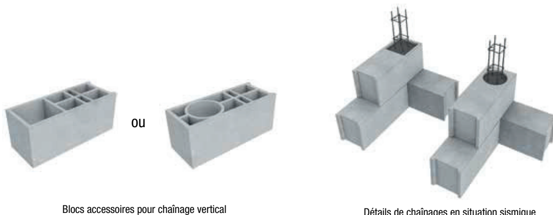
Détails de chaînages en situation sismique
